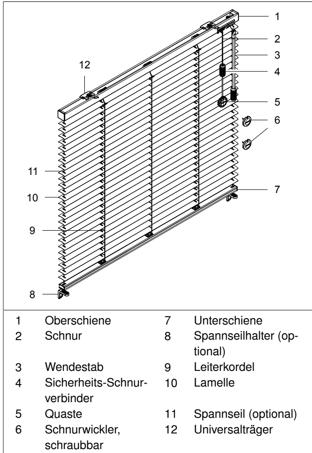
Abb. 1: Jalousie Select S mit Schnur/Stab
