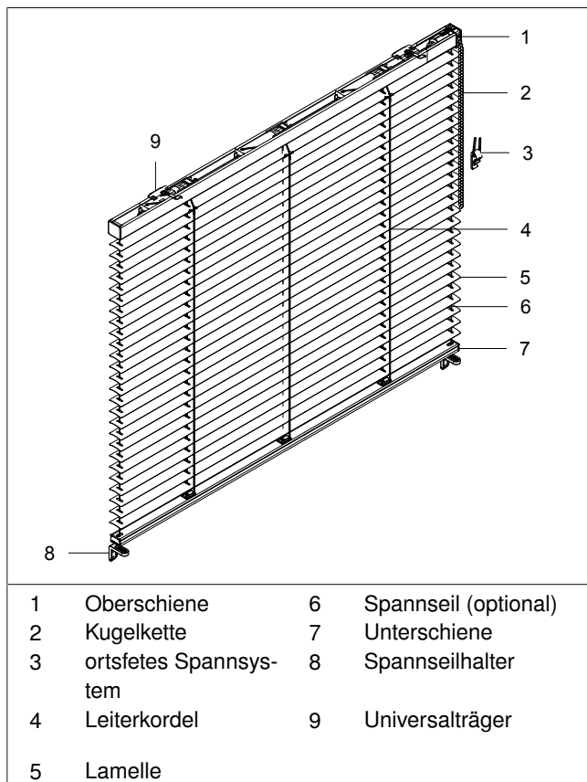
Abb. 1: Jalousie Select S mit Kugellkette
