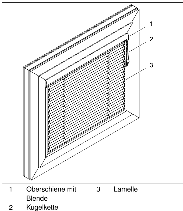
Abb. 1: Teileübersicht Glasleisten-Jalousie
