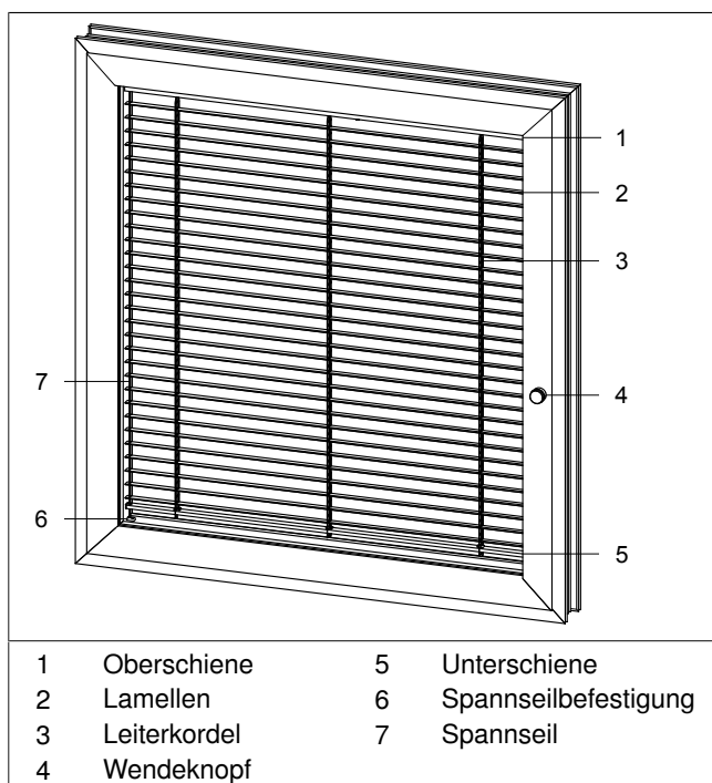
Abb. 1: Verbund-Jalousie M mit Wendeknopf
