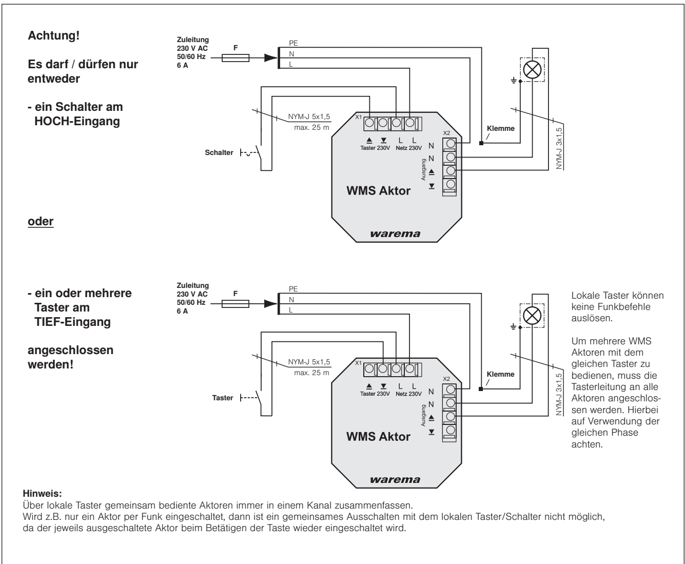
Abb. 3 Anschlussbeispiel Licht
