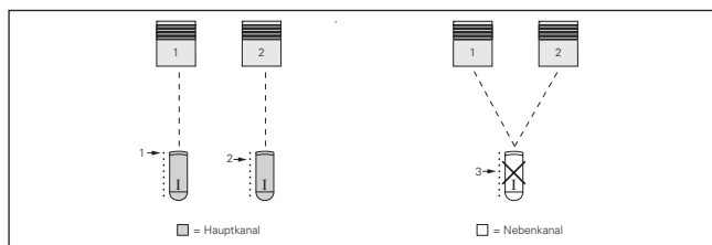
Abb. 3 Nebenkanäle in Empfänger 1 und 2 sollen gelöscht werden.
