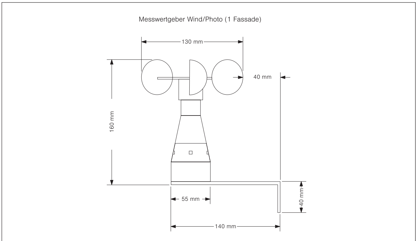
Abb. 2 Abmessungen
