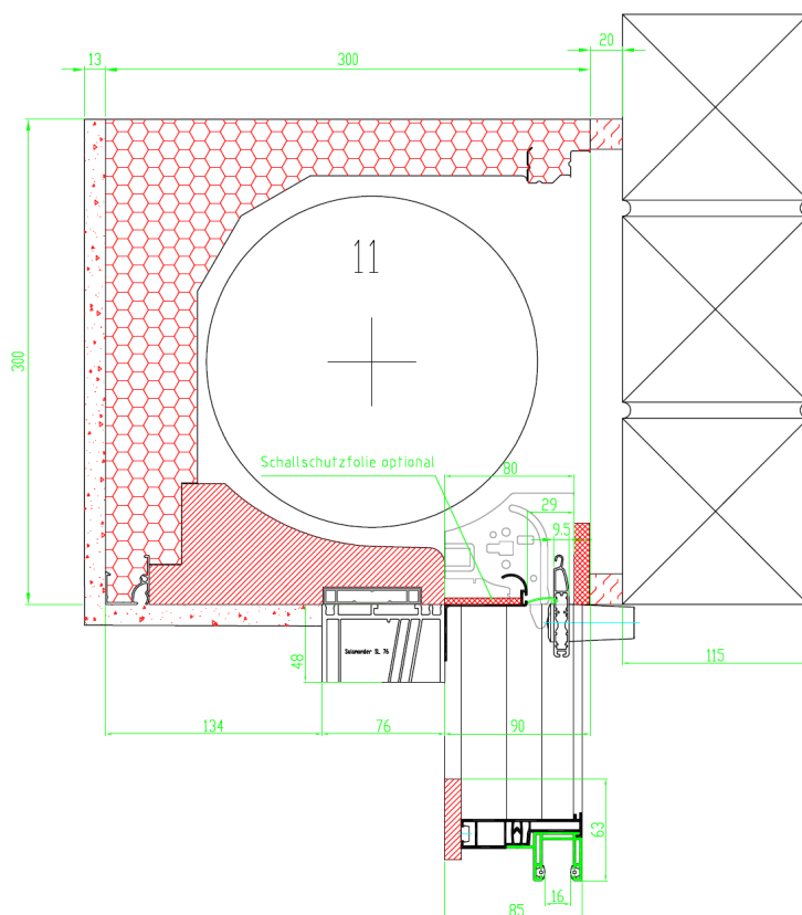
Bild 1 Schnittzeichnung (Grundsatzdetail, Ausführung ohne Schallschutzfolie, simulierte Klinkerfassade mit d = 70 \text{ mm} )
