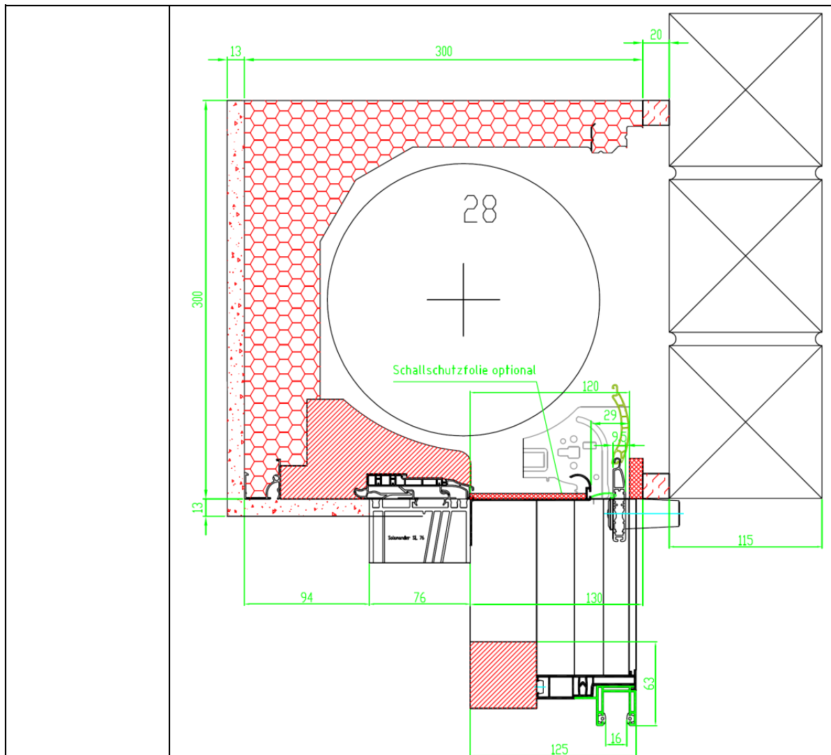
Beurteilung der Variante ohne Schallschutzfolie und simulierte Klinkerfassade mit d = 70 \text{ mm}
