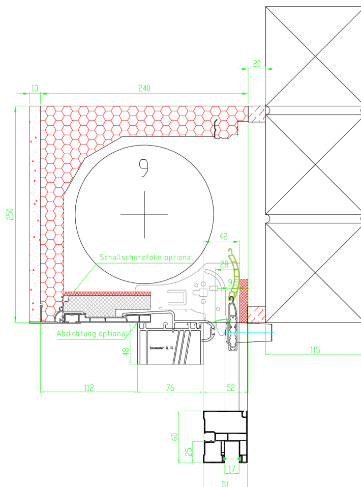
Bild 1 Schnittzeichnung (Grundsatzdetail, simulierte Klinkerfassade mit d = 70 mm, Ausführung mit Schallschutzfolie, ohne Abdichtung zum Fensterrahmen)
