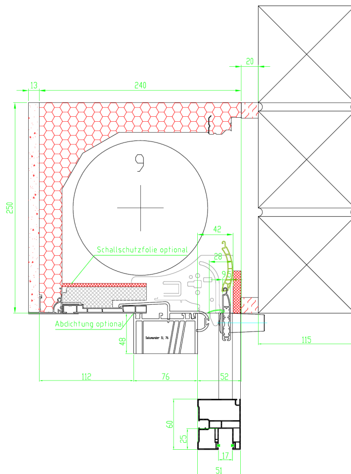
Bild 1 Schnittzeichnung (Grundsatzdetail, simulierte Klinkerfassade mit d = 70 mm, Ausführung ohne Schallschutzfolie, Anschluss an Fensterrahmen abgedichtet)
