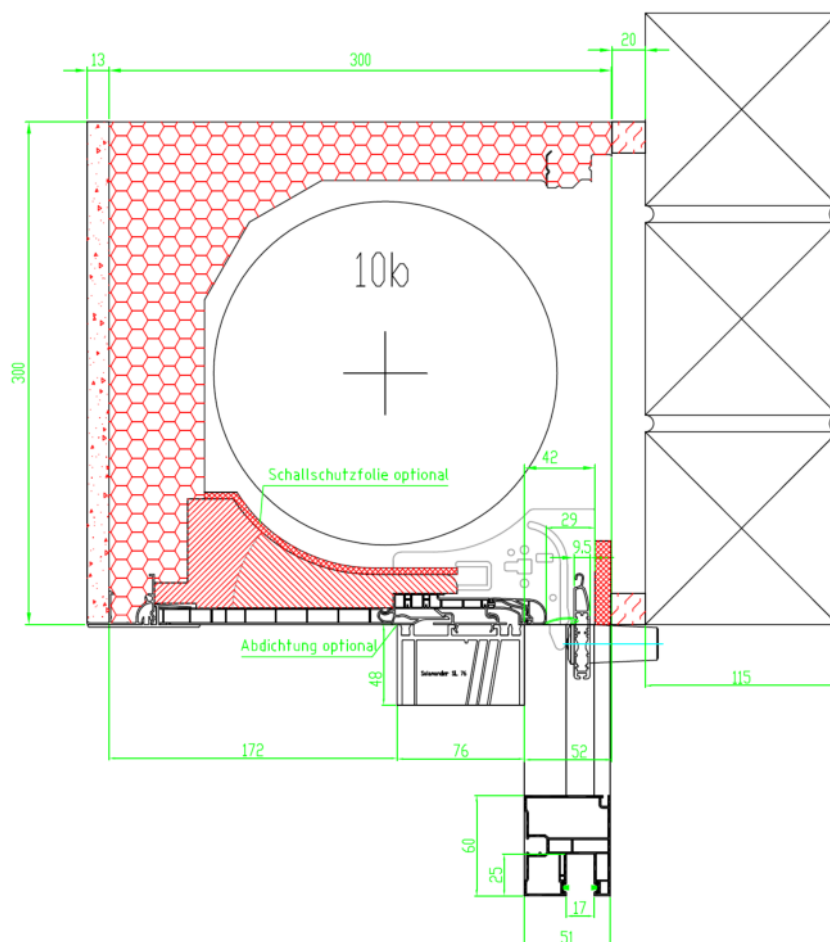
Bild 1 Schnittzeichnung (Grundsatzdetail, Ausführung mit Schallschutzfolie, Anschluss an Fensterrahmen abgedichtet, simulierte Klinkerfassade mit d = 70 \text{ mm} )
