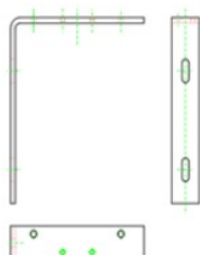
Typ 71 für bauseitigen Schacht
