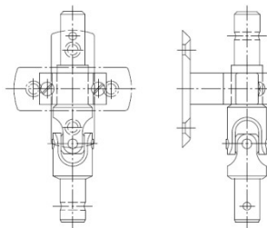
Rohrlager mit Kreuzgelenk
